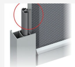
Ritssysteem voor een optimale opspanning van het doek
